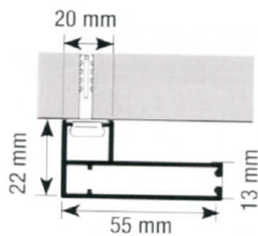
vodící profil
